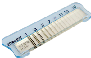
双丝像质计
