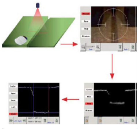
间隙检测
