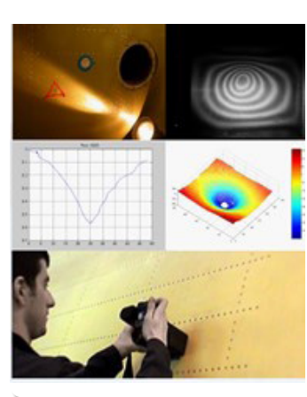
凹坑检测
