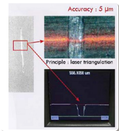
划痕检测
