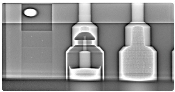
端塞焊缝检测
