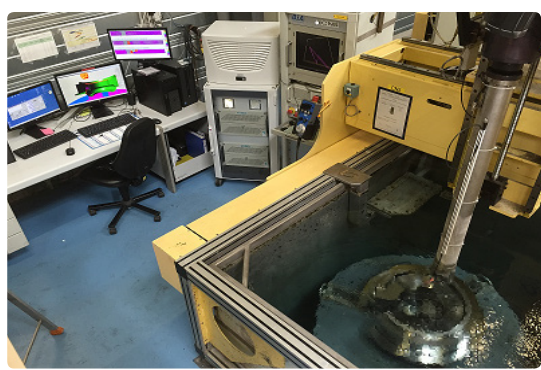
水浸检测系统集成
