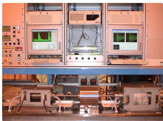
管/棒材检测系统集成
